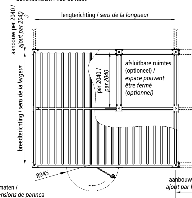
bovenaanzicht / vue de haut
