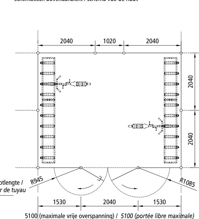
aanbouw per gootlengte / ajout par longueur de tuyau
